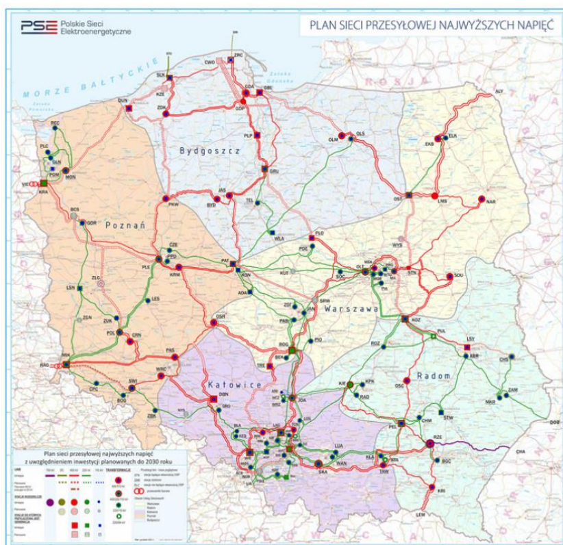
Rys. 11 Schemat Krajowego Systemu Przesyłowego (KSE)
