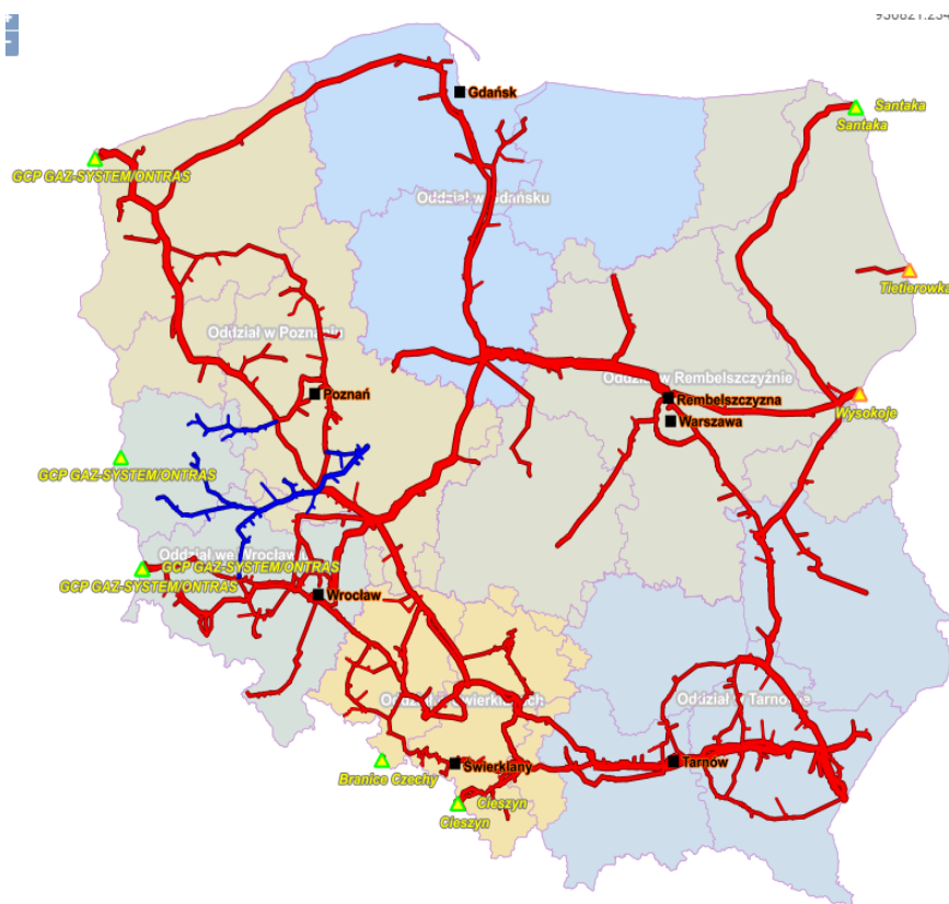
Rys. 12 System gazociągów przesyłowych na terenie Polski
