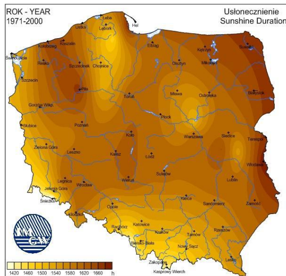
Rys. 6 Średnioroczne usłonecznienie
